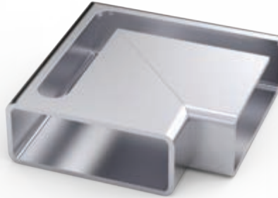
83361 80x30 Önden Kanallı Dirsek 90° 80x30 Front Channel Elbow 90° عكس مع قناة امامية 90 درجة 80*30
